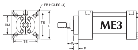
8.00" - 12.00" bores
