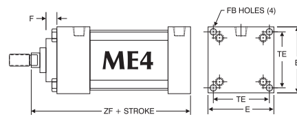
8.00" - 12.00" bores
