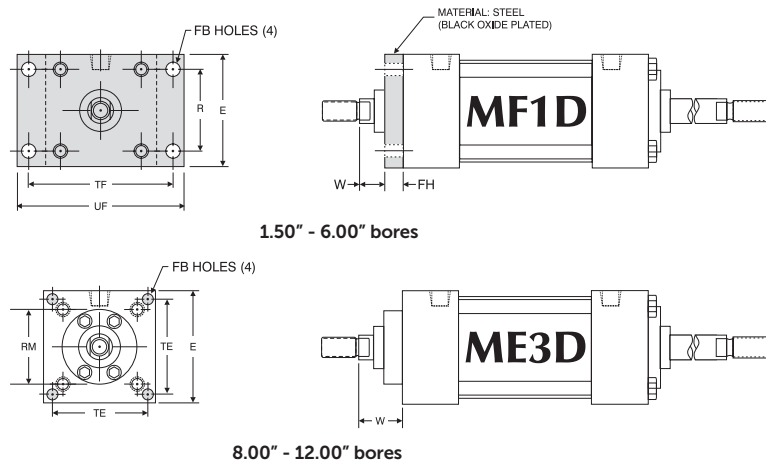
8.00" - 12.00" bores
